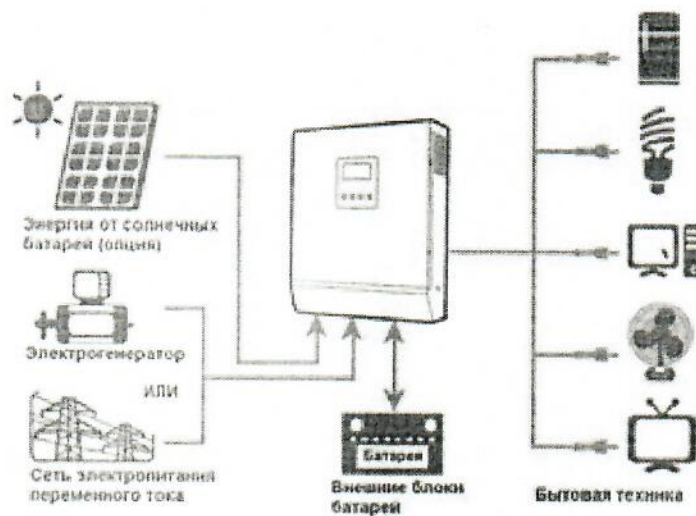
Рис. 1 Гибридная система электропитания
